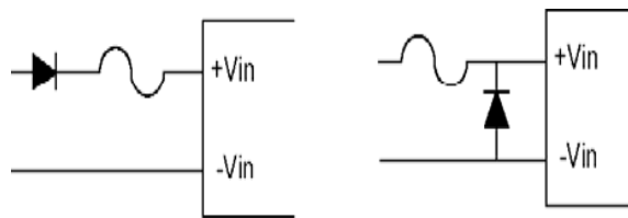
图(16) 输入反向保护以及过流保护
