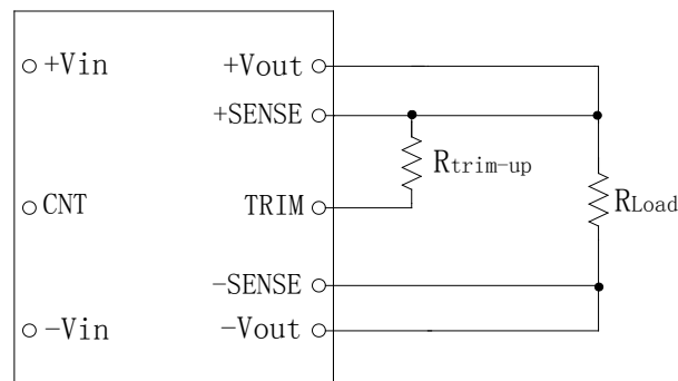
图(18) 输出电压上调节示意图
