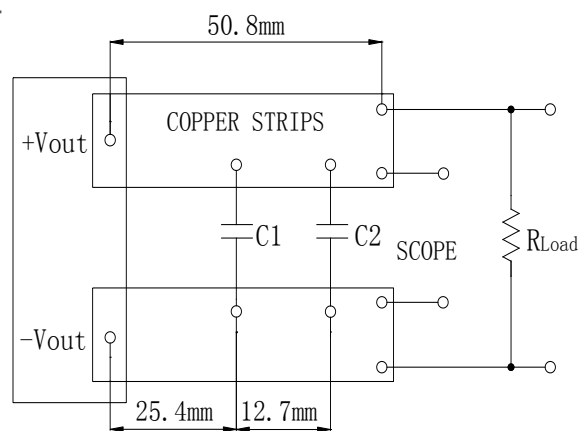
图(17) 输出纹波与噪声测试示意图
