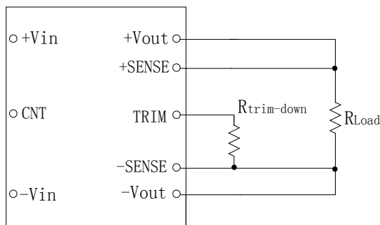
图(19) 输出电压下调示意图
