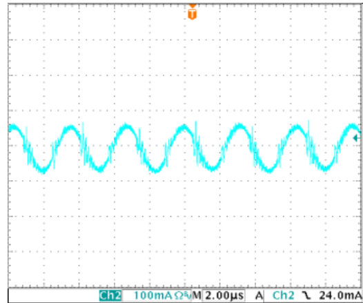
图(11) 反灌杂音电流波形（输入额定电压满载）
