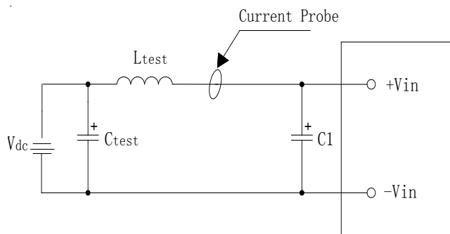
图(15) 输入反射纹波电流测试示意图
