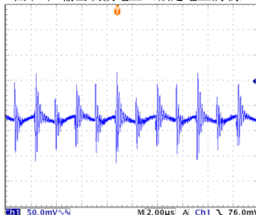
图(12) 输出纹波电压 (额定电压满载)
