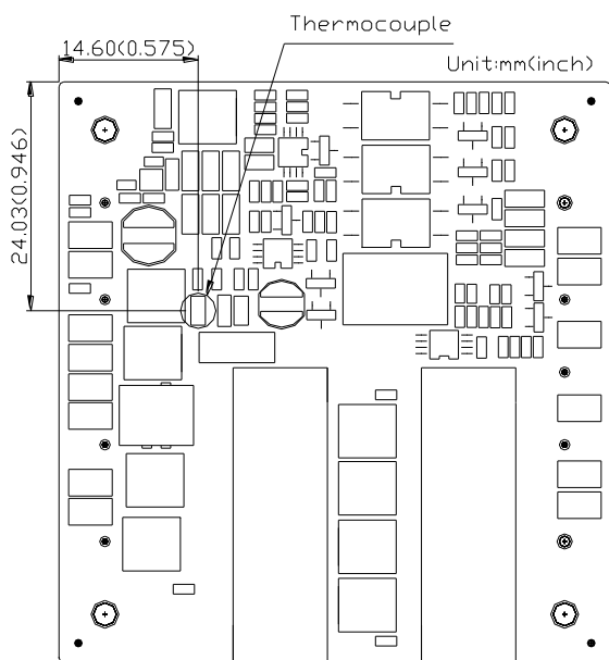
图(24) 温度测试点
