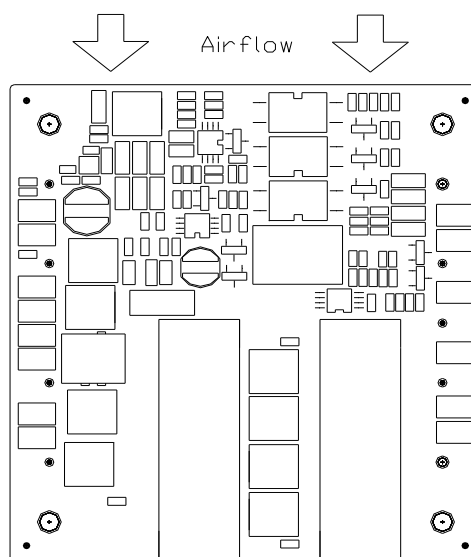
Top View 图(23) 散热方式示意图
