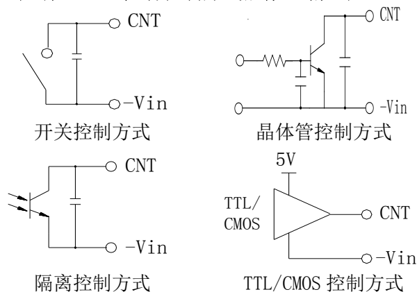
图(14) CNT 电路图
