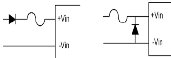
图(16) 输入反向保护以及过流保护
