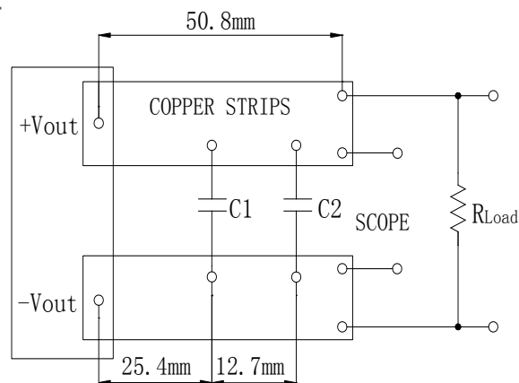
图(17) 输出纹波与噪声测试示意图
