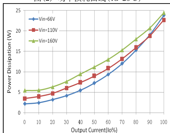
图(2) 功率损耗曲线 (Ta=25°C)
