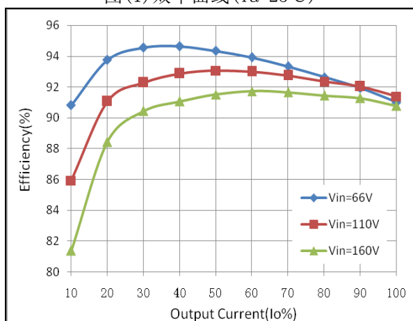
图(1) 效率曲线 (Ta=25°C)
