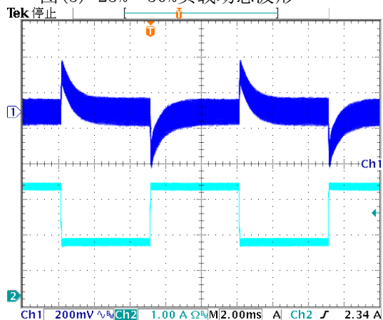
图(5) 25%~50%负载动态波形
