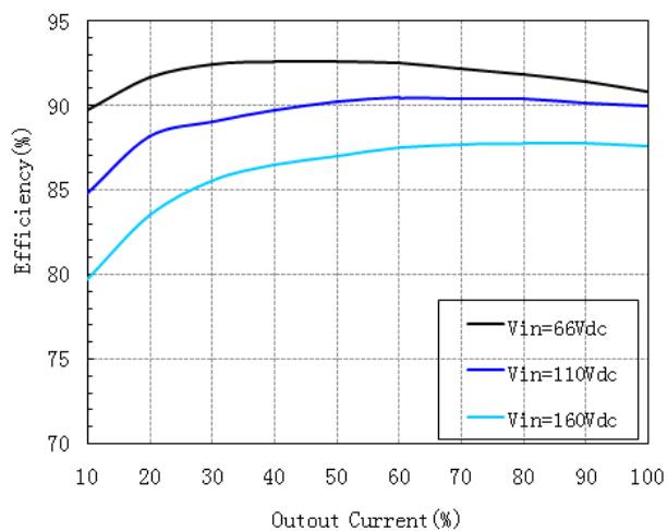
图(1) 效率曲线 (25℃)
