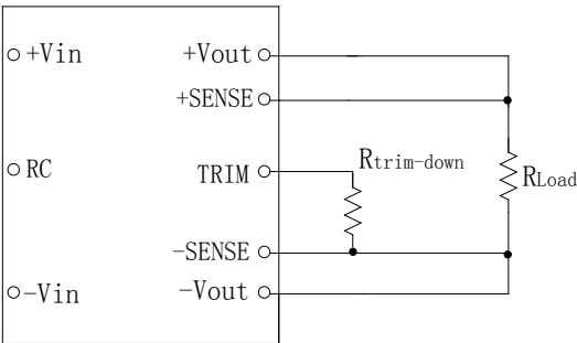
图 (10) 输出电压下调节示意图
