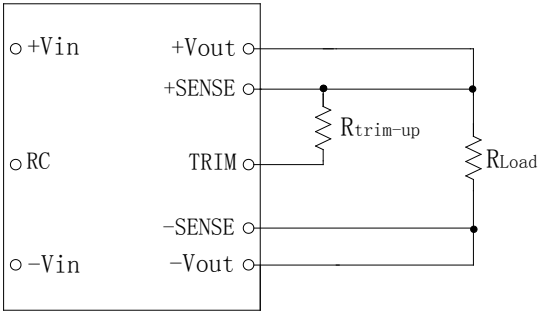
图 (9) 输出电压上调节示意图
