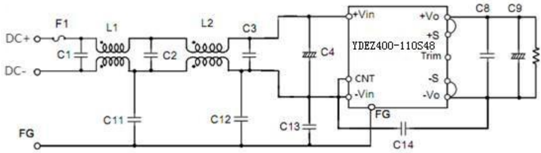
图 (7) 基本使用电路
